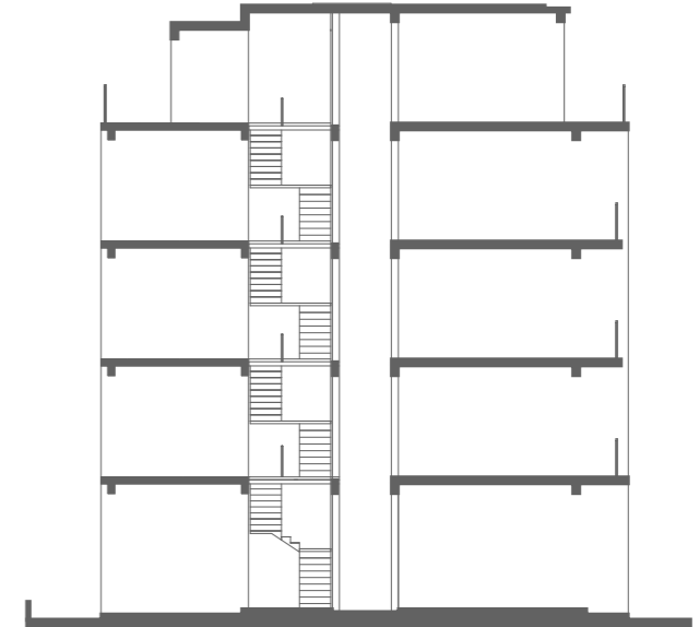
Mặt cắt
