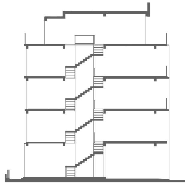
Mặt cắt
