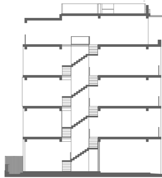
Mặt cắt
