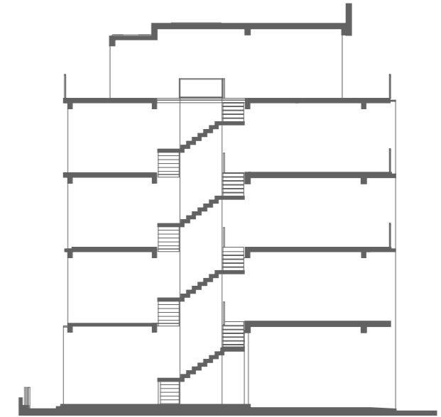
Mặt cắt
